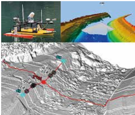
マルチビーム測深機による深浅測量
